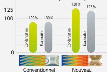
Efficacité des échanges thermiques (%)
