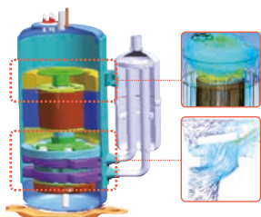
Optimisation du retour d'huile et adoption d'un système de séparation d'huile
